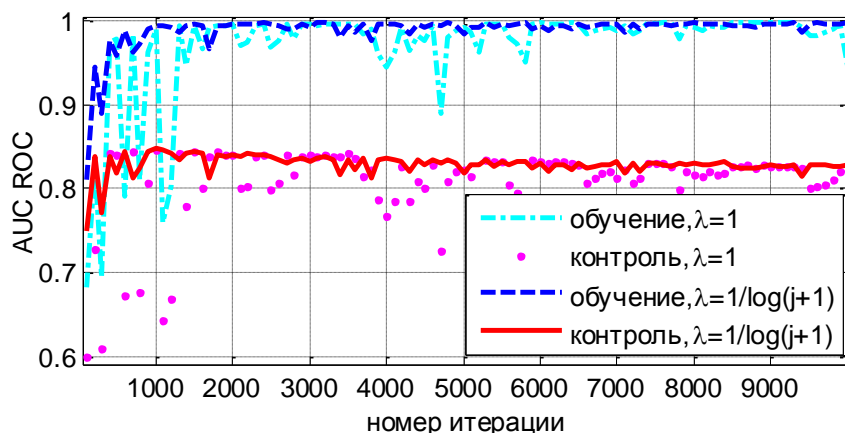
Рис. 1. Качество при настройке простейшего перцептронного алгоритма.
