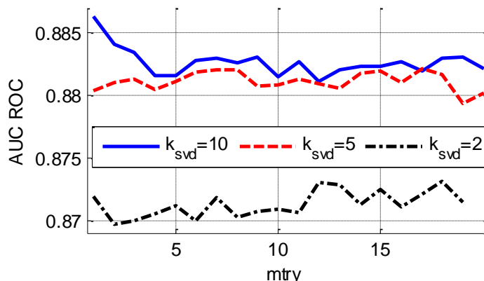
Рис. 9. Зависимость качества от параметра mtry случайного леса.
